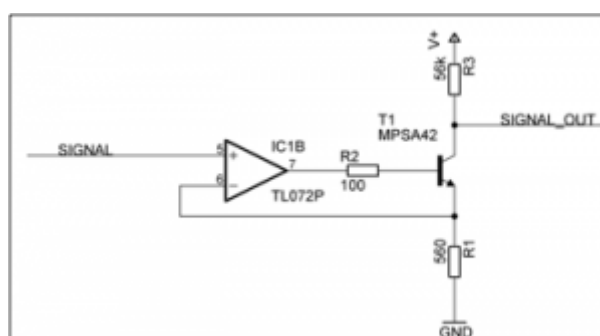
Obr. 8: Koncový stupeň VN zosilňovača
