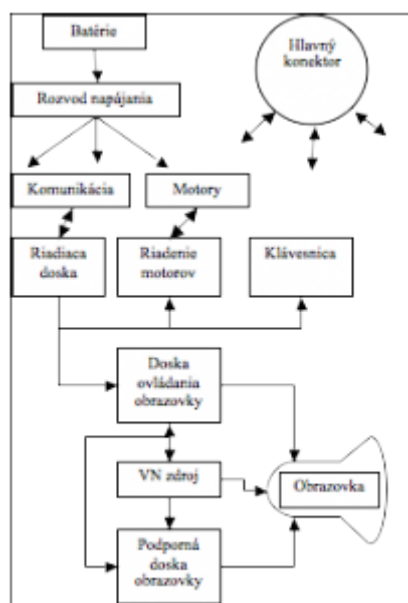
Obr.4: Bloková schéma robota
